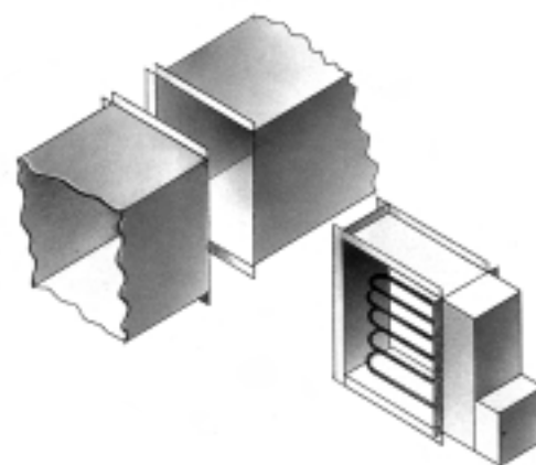
FIG. 5 - FLANGE TYPE
