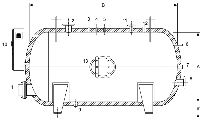
FIG. 5 - TYPE HC CALORIFIER
